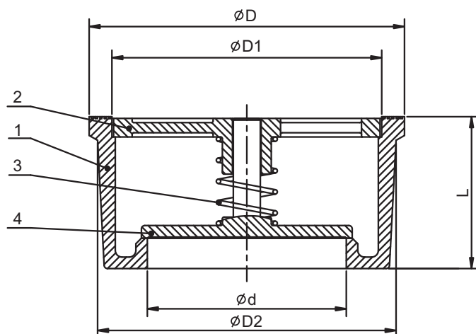
DN125-200
