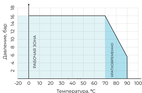
Диаграмма зависимости «Температура-Давление»
