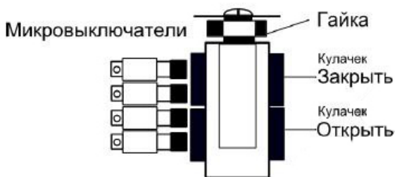
Рис. 5 - Настройка концевых выключателей
